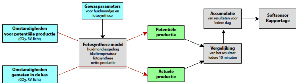
Fig. 8. Softsensor schema.
