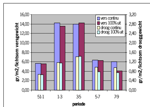
Grafiek 3.4: groei van vers- en drooggewicht/m2 per lichtevoelheid onder continue belichting of belichting 4 weken voor oogst uit in de tweede teelt
