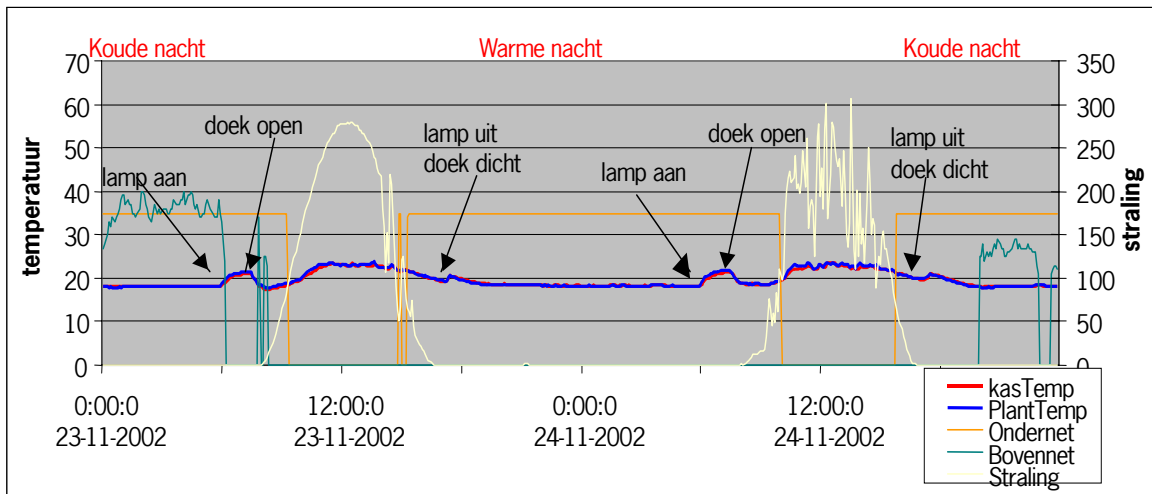
Grafiek 5.5: Klimaatoverzicht van de energiezuinige afdeling. In de grafiek zijn weergegeven de straling en ondernet, bovennet, kas-, en planttemperatuur.
