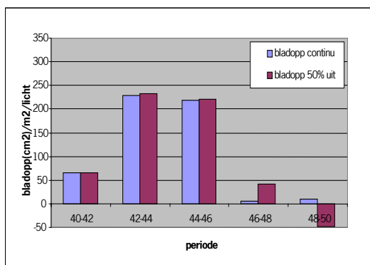
Grafiek 3.1: groei bladoppervlakte per m2 per lichtevoelheid in de eerste teelt
