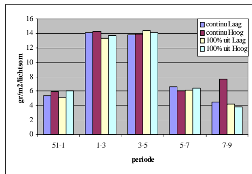
Grafiek 3.14: groei van het drooggewicht per lichthoeveelheid van planten in hoge en lage plantdichtheden (resp. 67 en 59 planten per m 2 ) onder twee belichtingsstrategieën
