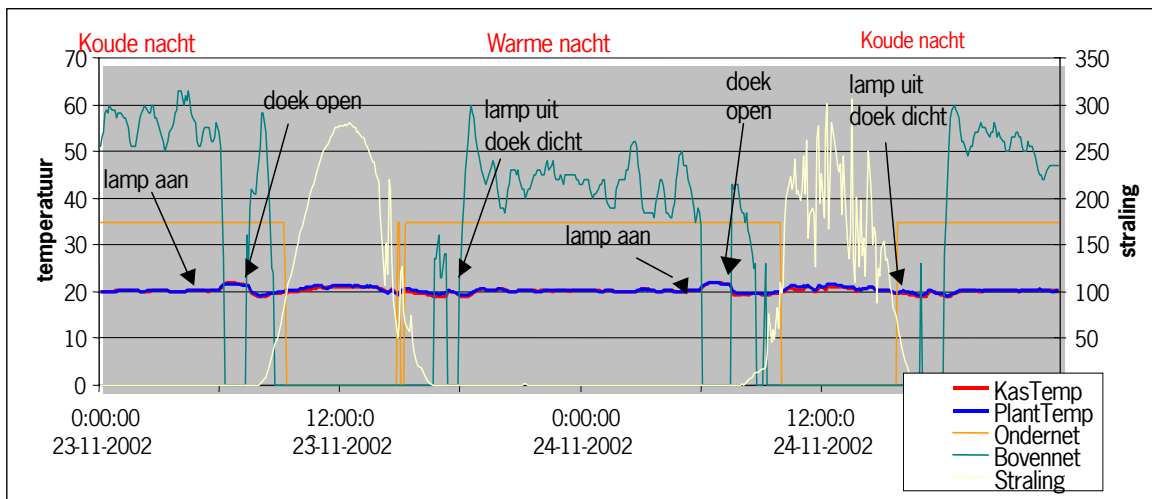
Grafiek 5.6: Klimaatoverzicht van de normale afdeling. In de grafiek zijn weergegeven de straling en ondernet, bovennet, kas- en planttemperatuur.
