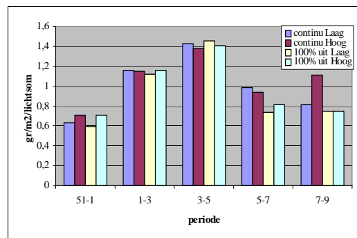
Grafiek 3.16: groei van het versgewicht per lichthoeveelheid van planten in hoge en lage plantdichtheden (resp. 67 en 59 planten per m 2 ) onder twee belichtingsstrategieën
