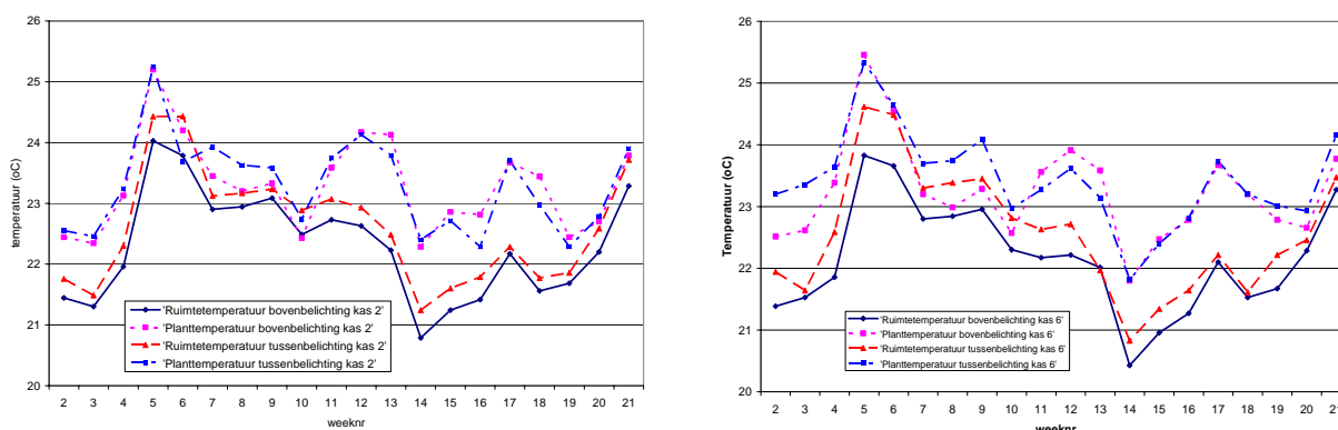
Figuur 4: Ruimte- en planttemperatuur gemiddeld per week in kasgedeelte met bovenbelichting en in kasgedeelte met tussenbelichting in respectievelijk kas 2 (links) en kas 6 (rechts).
