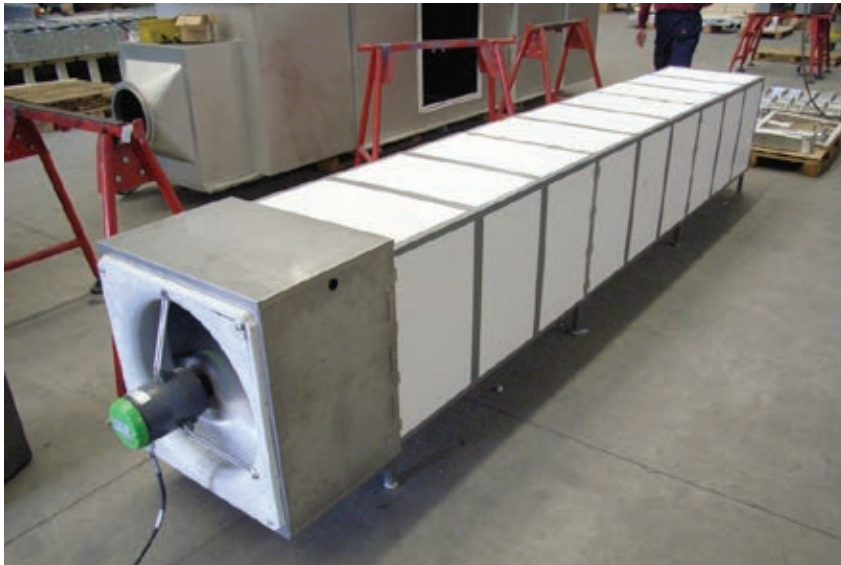
Figuur 4.1. FCA prototype 2 met kunststof omkasting en 4m lengte.
