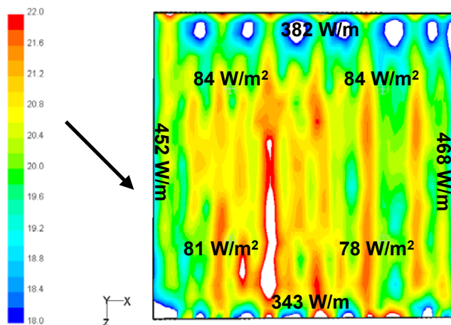
Figuur 20 Temperatuurverdeling bij een windsnelheid van 5 \text{ ms}^{-1} diagonaal op de kas bij een omgevingstemperatuur van 0 \text{ }^\circ\text{C} en een hemeltemperatuur van -10 \text{ }^\circ\text{C} waarbij er 100 \text{ Wm}^{-2} aan voelbare warmte aan het gewas wordt toegevoerd waarbij het gevelverwarmingsnet geregeld kan worden
