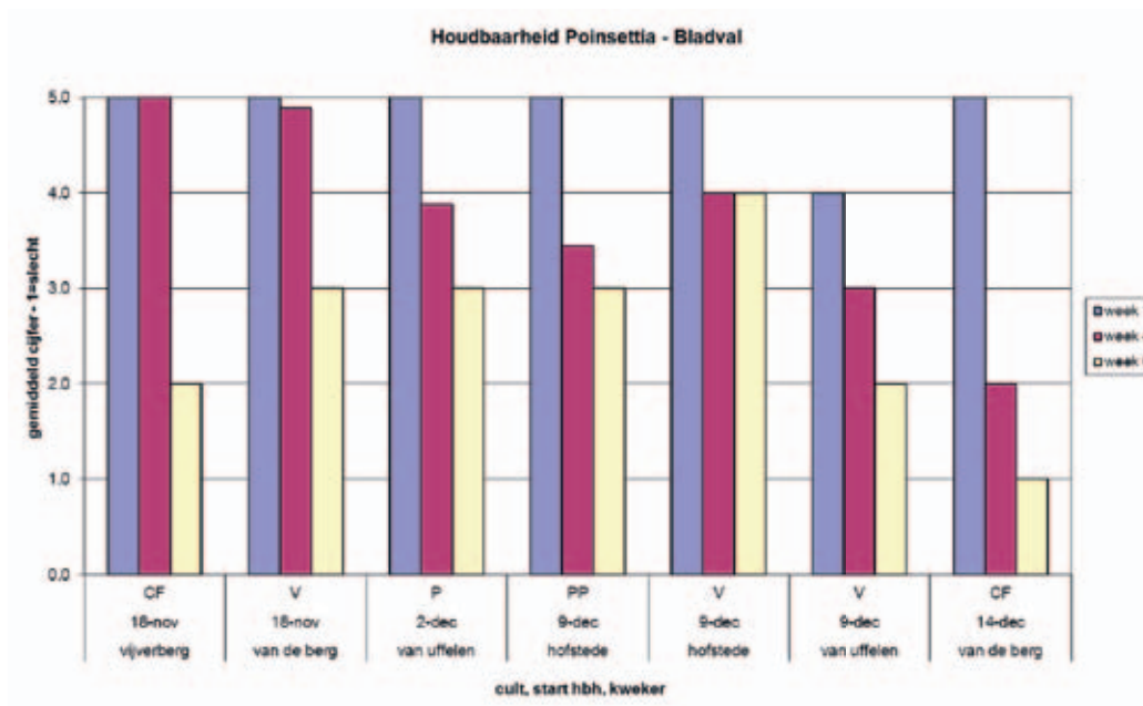
Figuur 3.3. Bladval als onderdeel van de houdbaarheid Poinsetta in 2009 met cultivar, einddatum en kweker, Cf=Christmas feeling, V=Viking, P= Premium en PP=Premium Polar na 1, 4 en 6 weken in uitbloeirimte.
