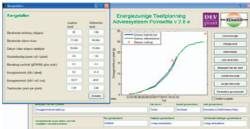
Figuur 3.5. Scenarioberekening met een vervoegd begin van de korte dag op 21 augustus (blauw, laatste run), vergeleken met een normaalteelt met natuurlijke korte dag (groen=natuurlijke korte dag, referentierun).
